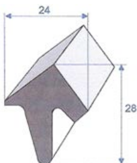
Réf. 7516 082 EPDM Cellulaire noir rouleau de 25 m
