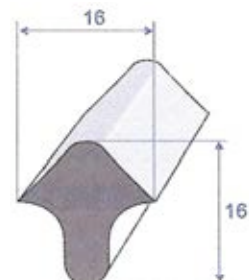
Réf. 7526 471 EPDM Cellulaire noir rouleau de 25 m
