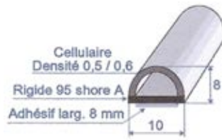
Réf. 6879 552 EPDM bi-durété noir adhésivé rouleau de 100 m
