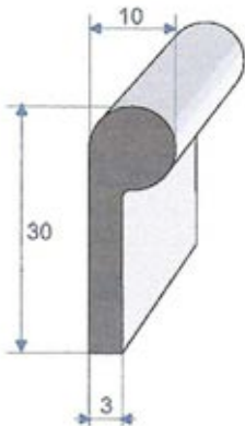
Réf. 7465 023 EPDM Cellulaire noir rouleau de 25 m
