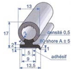
Réf. 7386 506 EPDM bi-durété noir adhésivé rouleau de 40 m
