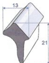
Réf. 7531 473 EPDM Cellulaire noir rouleau de 25 m
