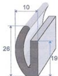
Réf. 7480 041 EPDM Cellulaire noir rouleau de 25 m
