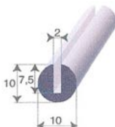
Réf. 1813 000 EPDM Cellulaire noir rouleau de 25 m
