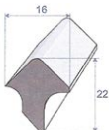
Réf. 7491 065 EPDM Cellulaire noir rouleau de 25 m
