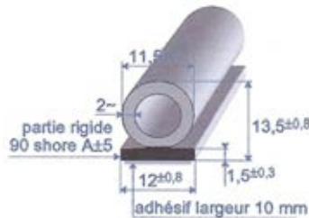
Réf. 7387 733 adhésivé Réf. 7387 833 sans adhésif EPDM bi-durété noir rouleau de 50 m
