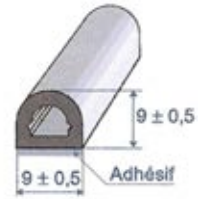
Réf. 6877 567 EPDM Cellulaire noir adhésivé rouleau de 50 m
