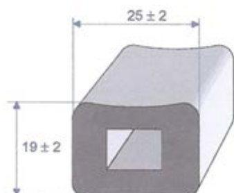
Réf. 7471 031 EPDM Cellulaire noir rouleau de 25 m
