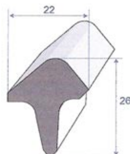
Réf. 7496 067 EPDM Cellulaire noir rouleau de 25 m
