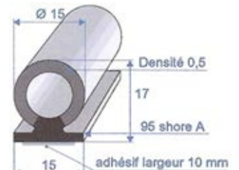
Réf. 7384 492 EPDM bi-durété noir adhésivé rouleau de 50 m
