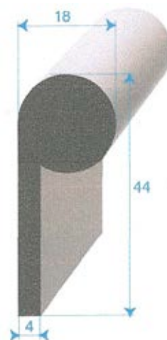
Réf. 1885 000 EPDM Cellulaire noir rouleau de 25 m
