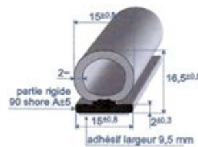
Réf. 7385 732 adhésivé Réf. 7385 832 sans adhésif EPDM bi-durété noir rouleau de 50 m
