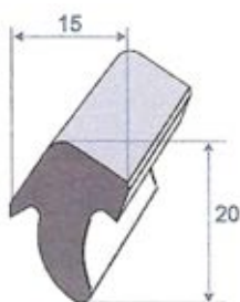
Réf. 7511 079 EPDM Cellulaire noir rouleau de 25 m
