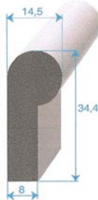
Réf. 1884 000 EPDM Cellulaire noir rouleau de 50 m
