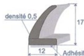
Réf. 6887 621 EPDM Cellulaire noir adhésivé rouleau de 60 m
