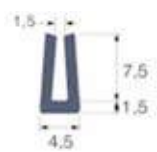
Réf. 7156 492 SEBS 65 shore A coloris au choix* rouleau de 50 m
