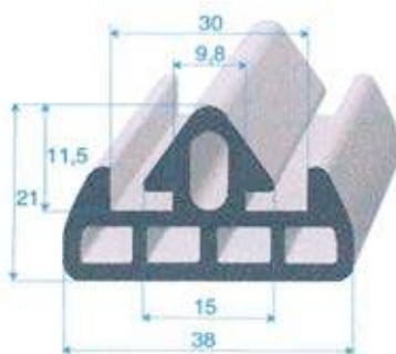
Réf. 1828 000 EPDM noir 70 shore A ± 5 rouleau de 25 m
