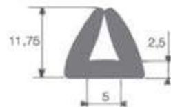
Réf. 7180 015 SBR noir 60 shore A \pm 5 rouleau de 50 m
