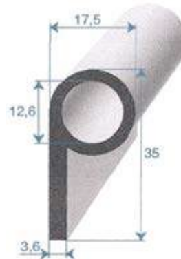
Réf. 1852 000 EPDM noir 70 shore A ± 5 rouleau de 50 m
