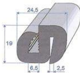
Réf. 7232 314 EPDM noir 70 shore A ± 5 rouleau de 25 m
