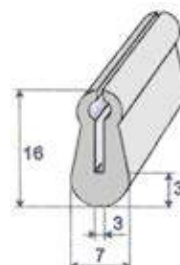
Réf. 7070 223 TPE gris 60 shore A ± 5 rouleau de 50 m
