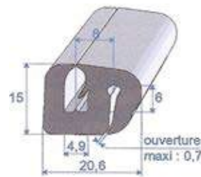
Réf. 7229 546 EPDM noir 70 shore A ± 5 rouleau de 30 m
