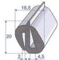
Réf. 7217 310 EPDM noir 80 shore A ± 5 rouleau de 25 m
