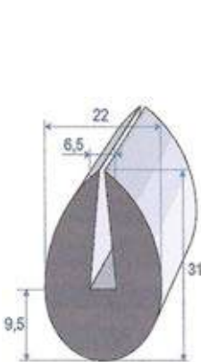
Réf. 7060 348 EPDM noir 70 shore A ± 5 rouleau de 20 m
