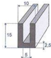
Réf. 7140 124 EPDM noir 70 shore A \pm 5 rouleau de 50 m
