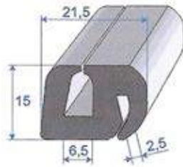
Réf. 7230 256 EPDM noir 70 shore A ± 5 rouleau de 30 m
