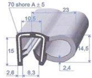
Réf. 6897 561 EPDM bi-durété noir + armature métal. A = 7 à 9 mm rouleau de 50 m
