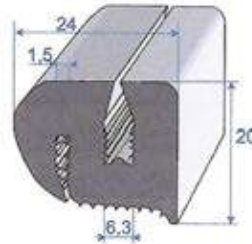
Réf. 7236 271 EPDM noir 70 shore A ± 5 rouleau de 20 m
