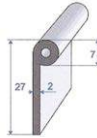
Réf. 7295 318 EPDM noir 60 shore A ± 5 rouleau de 50 m
