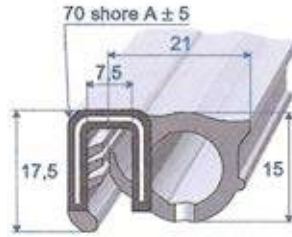
Réf. 6932 466 EPDM bi-durété noir + armature métal. A = 5 à 6 mm rouleau de 50 m
