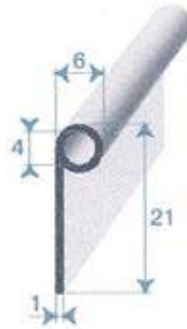
Réf. 1845 000 EPDM noir 70 shore A ± 5 rouleau de 50 m
