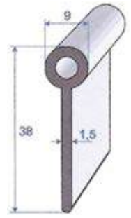
Réf. 7345 225 EPDM noir 75 shore A ± 5 rouleau de 50 m
