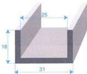
Réf. 1865 000 EPDM noir 70 shore A ± 5 rouleau de 25 m
