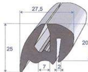
Réf. 7233 319 EPDM noir 70 shore A ± 5 rouleau de 30 m
