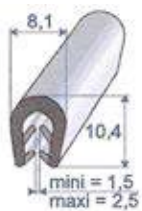
Réf. 6880 500 EPDM noir 95 shore A rouleau de 100 m
