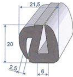
Réf. 7220 255 EPDM noir 70 shore A ± 5 rouleau de 30 m
