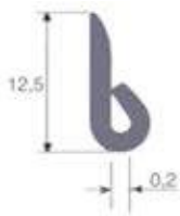
Réf. 7085 015 SBR noir 60 shore A ± 5 rouleau de 100 m
