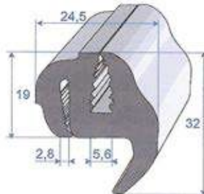
Réf. 7235 317 EPDM noir 70 shore A ± 5 rouleau de 20 m
