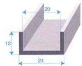
Réf. 1864 000 EPDM noir 70 shore A ± 5 rouleau de 50 m
