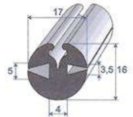
Réf. 7238 327 EPDM noir - 70 shore A ± 5 rouleau de 30 m clé adaptable : 7260 270
