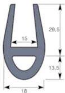
Réf. 7156 430 SEBS 65 shore A coloris au choix* - long. 2 m
