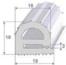
Réf. 7367 326 TPE gris 60 shore A ± 5 rouleau de 25 m
