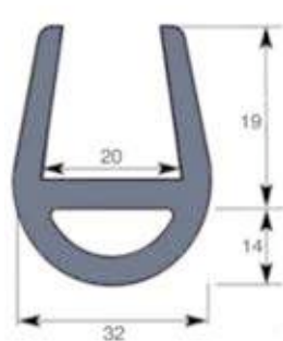
Réf. 7156 440 SEBS 65 shore A coloris au choix* - long. 2 m
