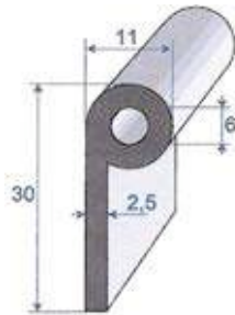
Réf. 7305 236 EPDM noir 70 shore A ± 5 rouleau de 50 m
