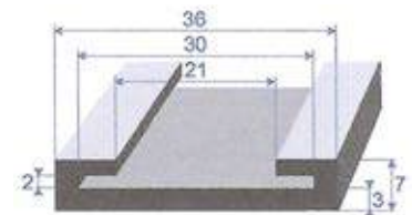
Réf. 7281 703 EPDM noir 70 shore A ± 5 rouleau de 50 m
